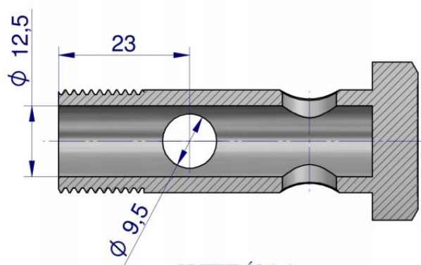
PRZEKRÓJ A-A
