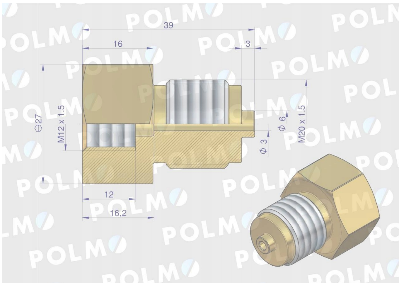
Złączka manometryczna gwint zewnętrzny M20x1.5 x gwint wewnętrzny M12x1.5 (mosiądz) POLMO
