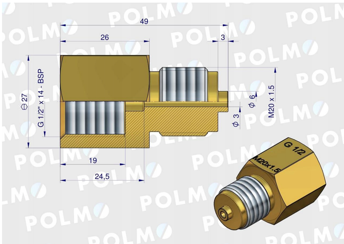
Złączka manometryczna gwint zewnętrzny M20x1.5 x gwint wewnętrzny G1/2" (mosiądz) POLMO
