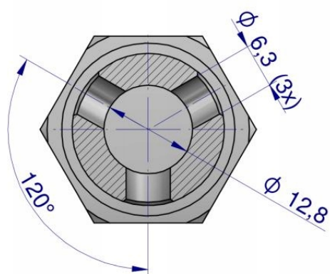
PRZEKRÓJ A-A
