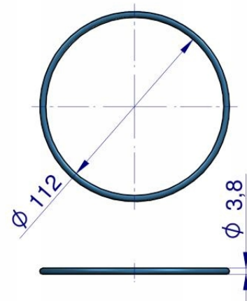
Pierścień segra W40 (2 szt.)
