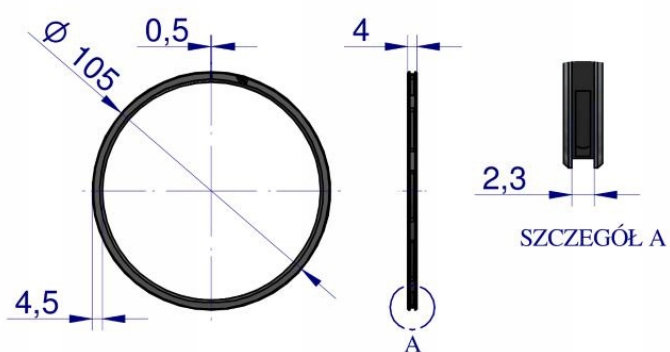
Pierścień olejowy
