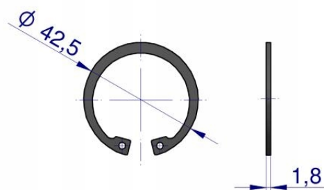
Pierścień segra W40 (2 szt.)
