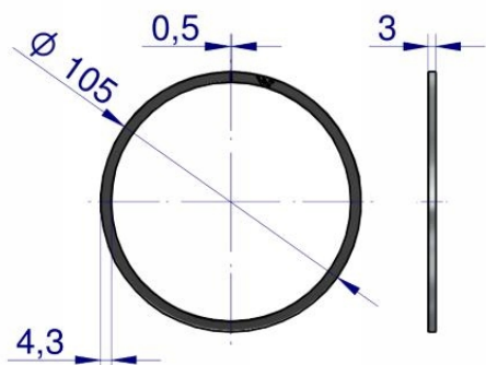
Pierścień uszczelniający tłoka chromowany
