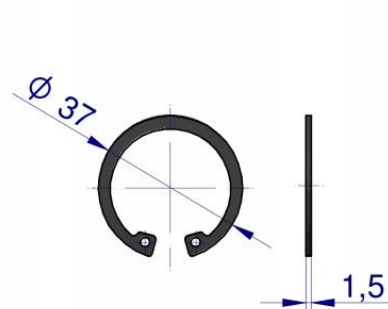
Pierścień segera W35 (2 szt.)
