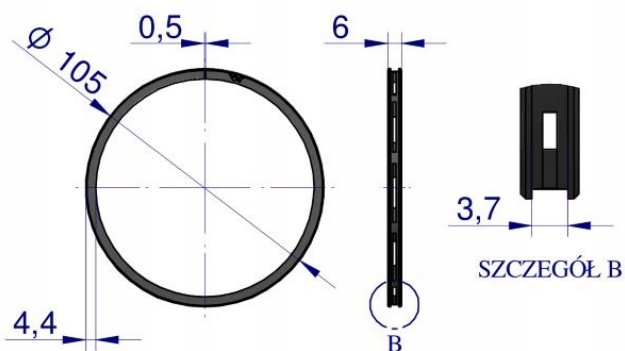
Pierścień olejowy
