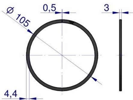
Pierścień uszczelniający tłoka (2szt.)
