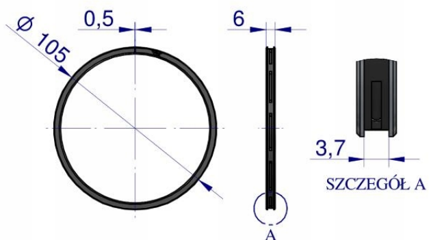
Pierścień olejowy chromowany
