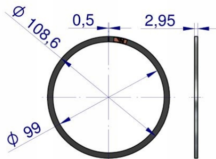
Pierścień uszczelniający tłoka chromowany
