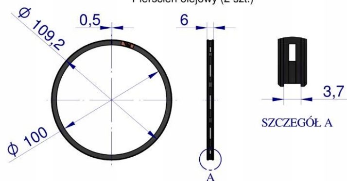
Pierścień olejowy (2 szt.)
