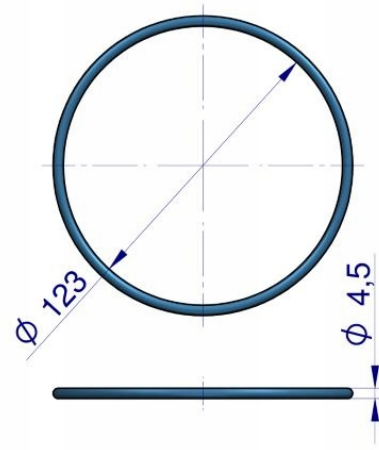
Oring uszczelniający tulei (2 szt.)
