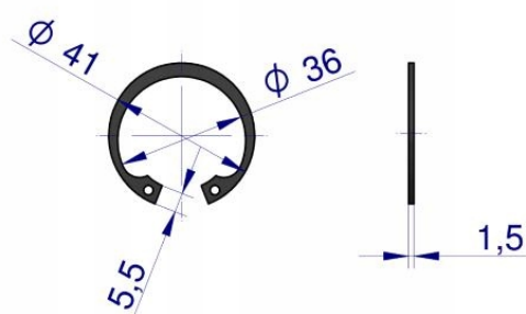
Pierścień segera ( 2 szt.)
