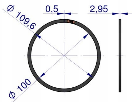
Pierścień uszczelniający tłoka (2 szt.)
