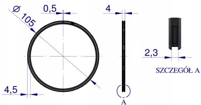
Pierścień olejowy
