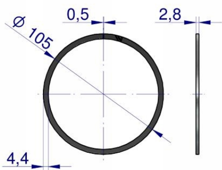
Pierścień olejowy
