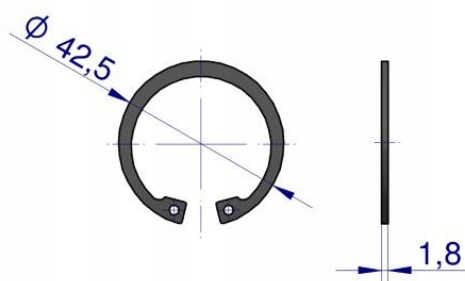
Pierścień segera W40 (2 szt.)
