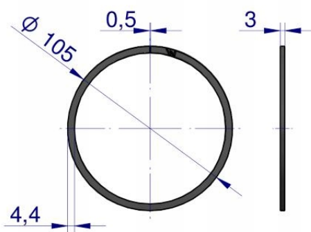
Pierścień uszczelniający tłoka
