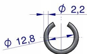
Pierścień zabezpieczający - 1x
