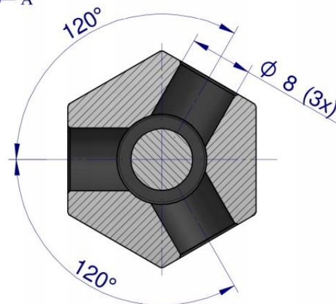
PRZEKRÓJ A-A
