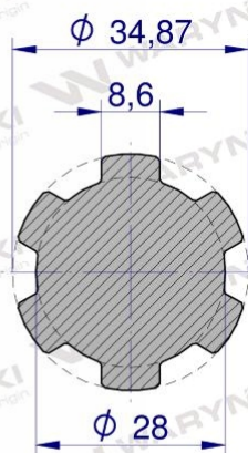
PRZEKRÓJ A-A
