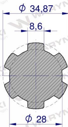
PRZEKRÓJ A-A
