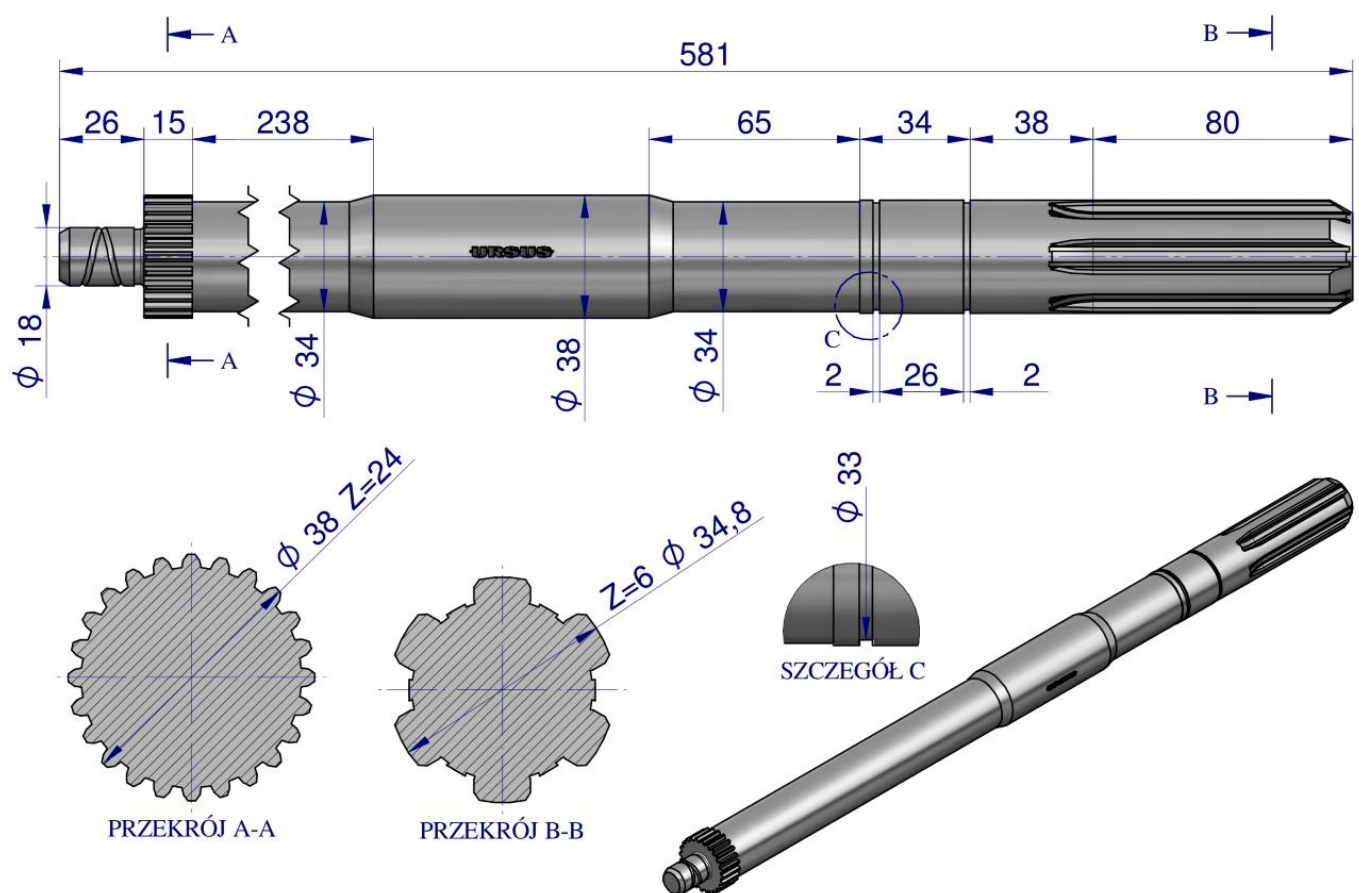
Wałek przekąźnika mocy II WOM C-360 ORYGINAŁ URSUS
