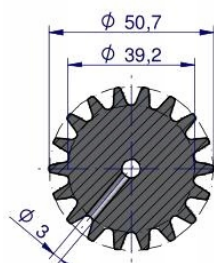
PRZEKRÓJ A-A
