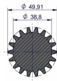
PRZEKRÓJ B-B
