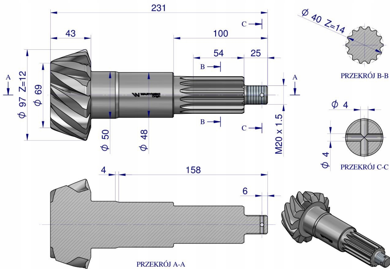
Walek atakujacy z kołem talerzowym C-385 80170989 WARYŃSKI
