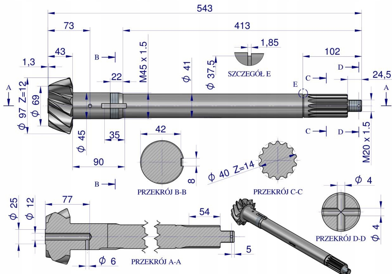
Walek atakujący z kołem talerzowym C-385 88170989 WARYŃSKI
