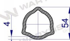
Rura wewnętrzna
