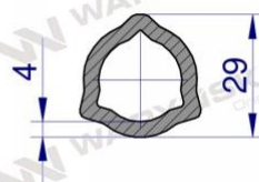
Rura wewnętrzna
