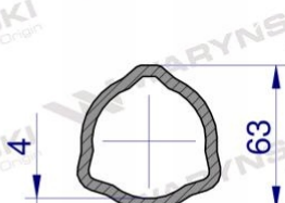
Rura zewnętrzna
