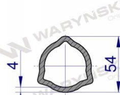
Rura wewnętrzna
