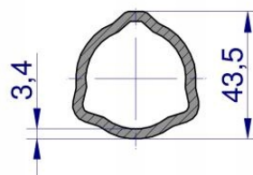
Rura zewnętrzna
