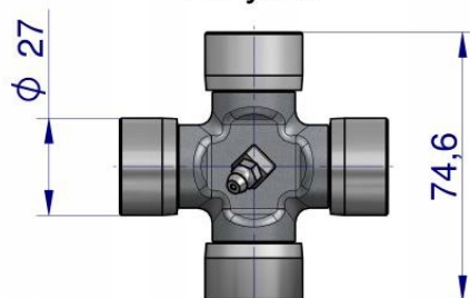
Krzyżak
