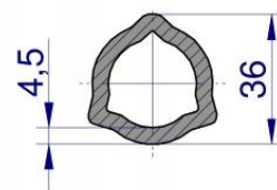
Rura wewnętrzna
