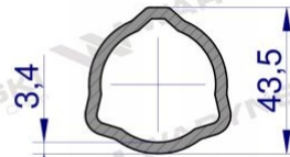
Rura zewnętrzna
