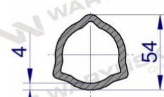
Rura wewnętrzna
