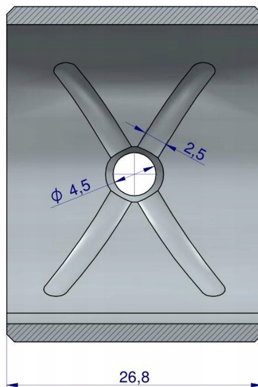
PRZĘKRÓJ A-A
