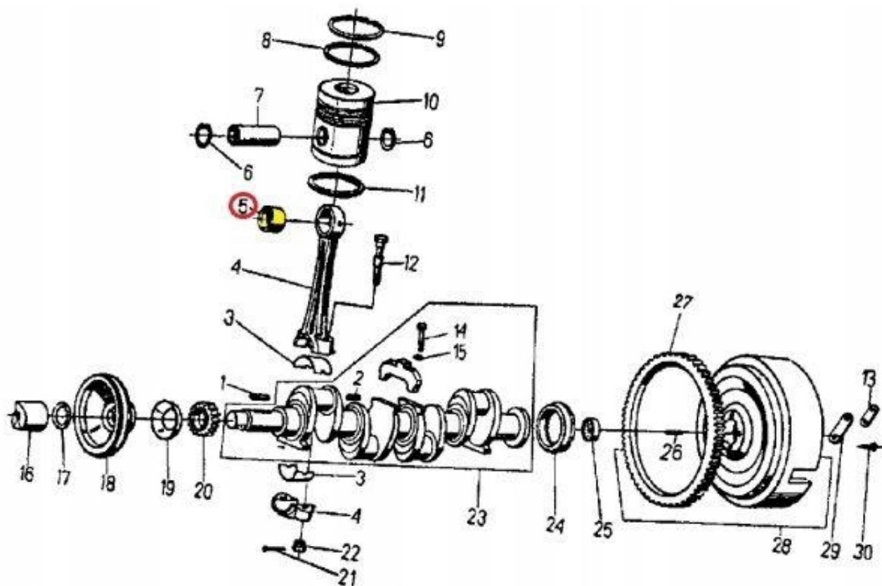
Tuleja korbowodu 950311 C 360 / Zetor (nominalna)
