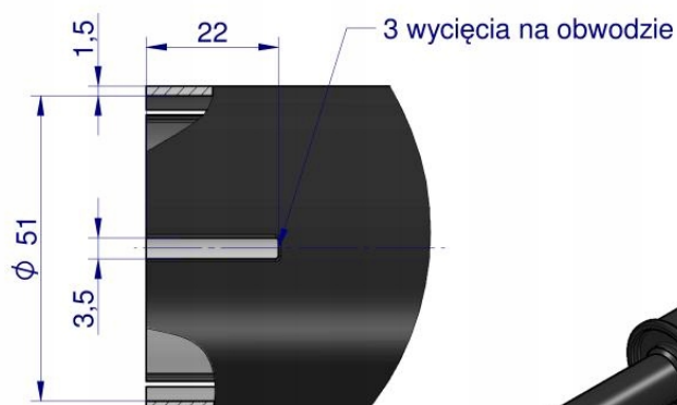
SZCZEGÓŁ A
