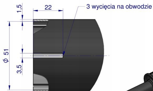
SZCZEGÓŁ A
