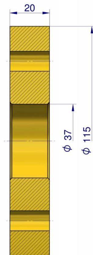
PRZEKRÓJ A-A
