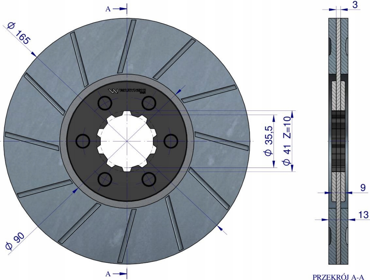
PRZEKRÓJ A-A
