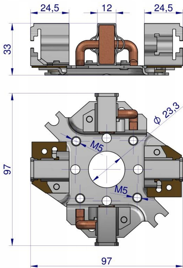
Szczotkotrzymacz
