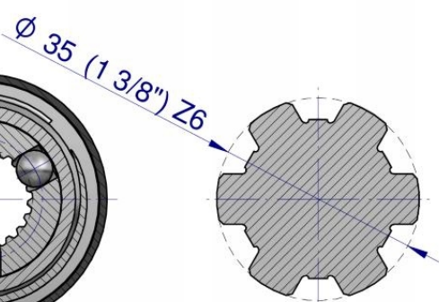
PRZEKRÓJ B-B 2:1
