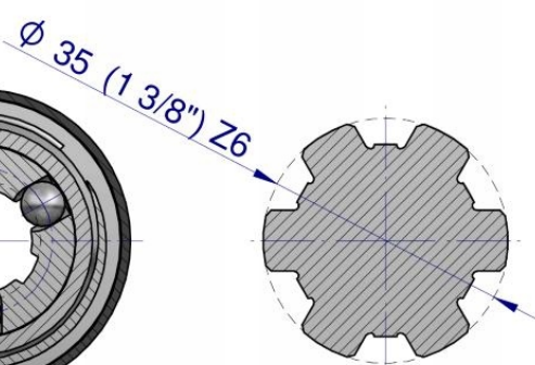
PRZEKRÓJ B-B 2:1
