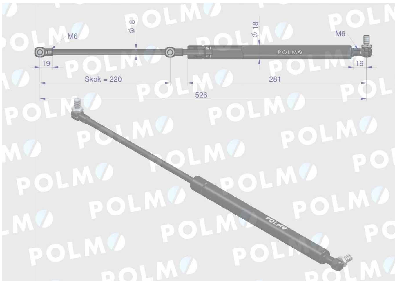
Siłownik szyby tylnej 10368917P ZETOR POLMO
