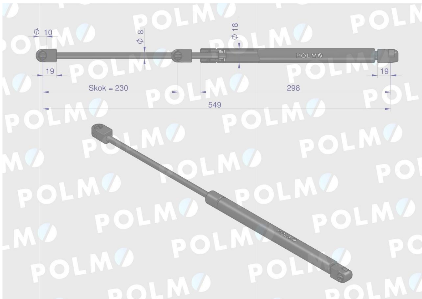
Siłownik szyby tylnej CASE IH POLMO
