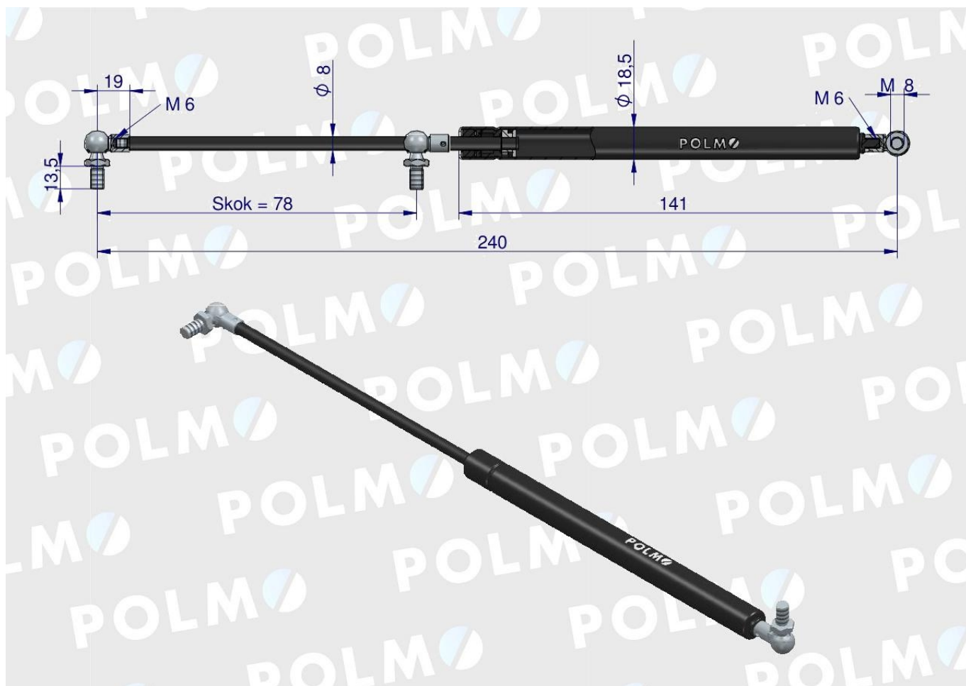
Siłownik szyby przedniej szyby drzwi CASE IH DEUTZ POLMO
