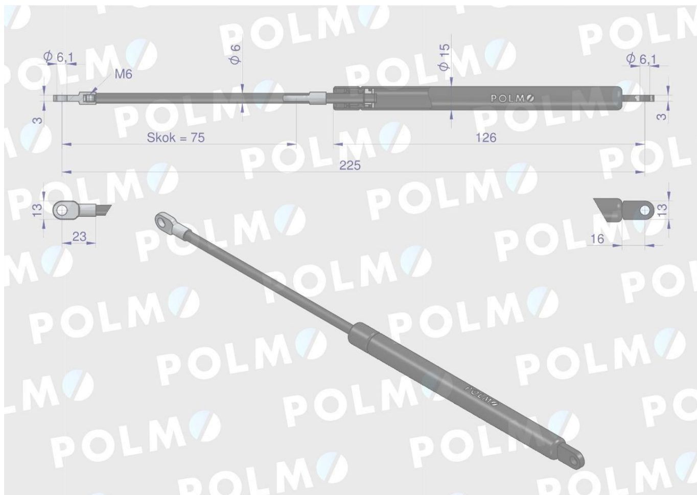
Siłownik szyberdachu CASE IH JOHN DEERE POLMO
