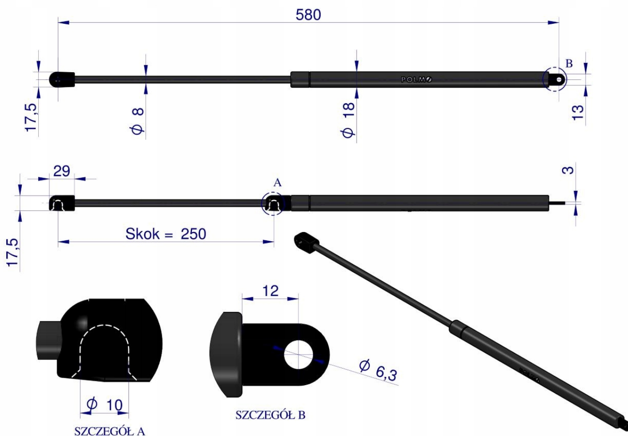
Siłownik podnoszenia maski New Holland 5166403 POLMO
