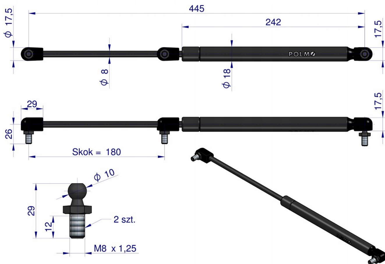
Siłownik podnoszenia maski New Holland 5177277 POLMO
