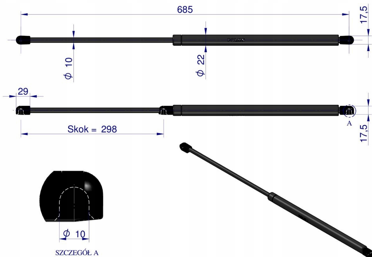
Siłownik podnoszenia maski New Holland 82011092 POLMO
