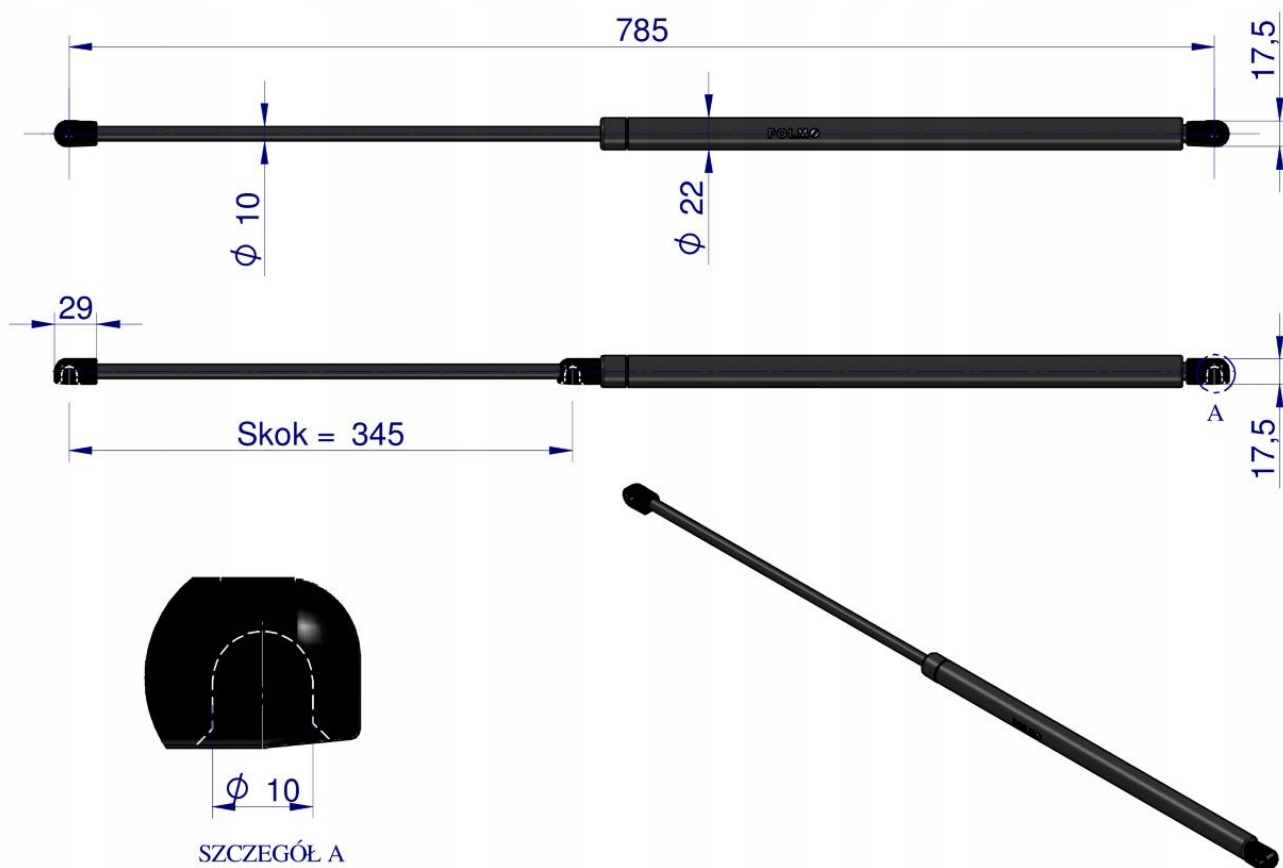
Siłownik podnoszenia maski John Deere RE63872 POLMO
