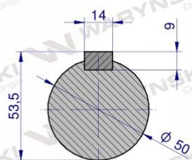
PRZĘKROJ A-A
