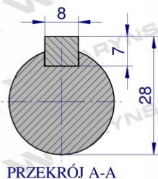
PRZEKRÓJ A-A
