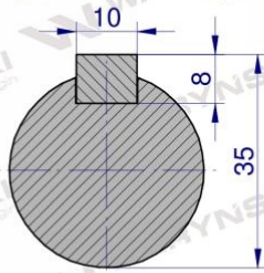
PRZEKRÓJ A-A
