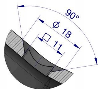
SZCZEGÓŁ B 3:1
