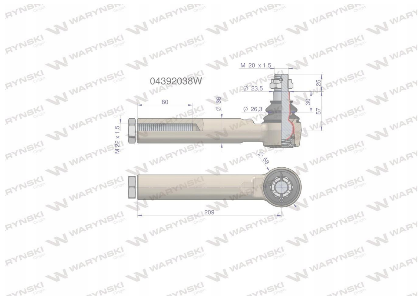
Przegub kierowniczy 04392038 Deutz; Renault; Valmet WARYŃSKI
