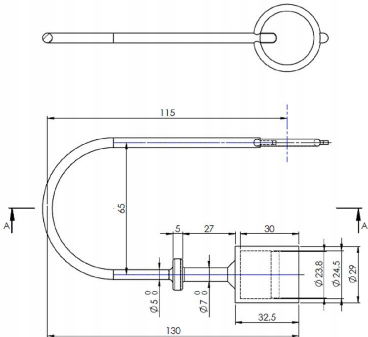
PRZEKRÓJ A-A
