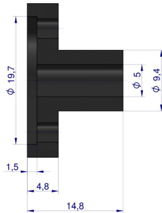
PRZĘKRÓJ A-A
