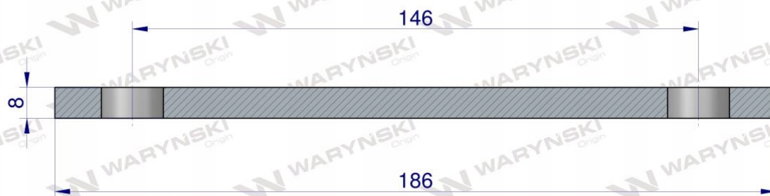
PRZEKRÓJ A-A
