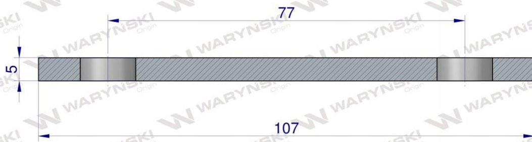
PRZĘKRÓJ A-A
