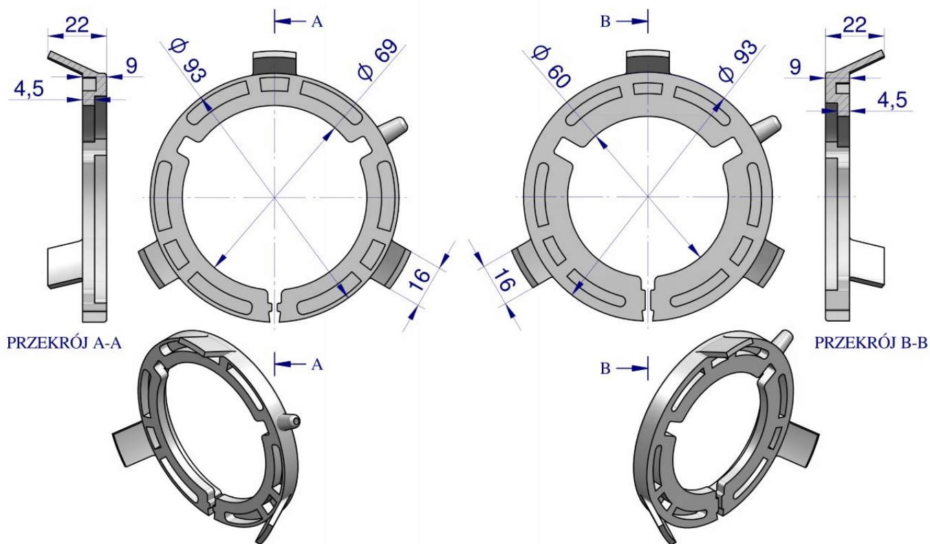
Pierścień zewnętrzny
